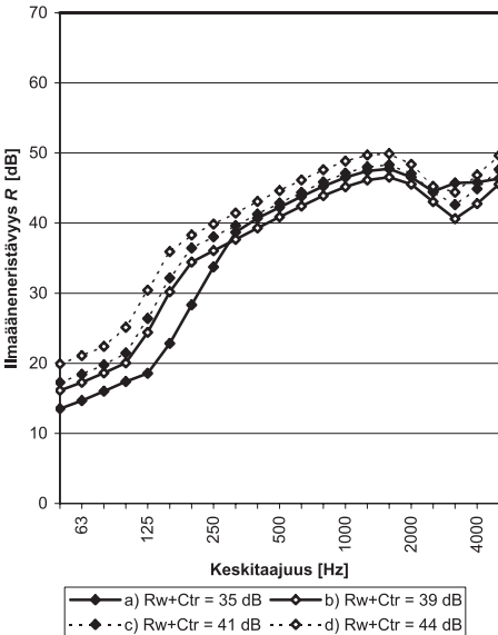
Kuva 6. Ulkoseinära- kenteen laskettuja ilmää- neristävyyksiä ja ilmääneneristyslukuja tie- liikennemelua vastaan R_w + C_{tr} . Perusrakenne on tuulensuojalevy, puurunko 150 mm k600 (vä- lissä mineraalivilla), sisäverhouslevy. Lasketut vaihtoehdot: a) tuulensuojakuitulevy, sisäver- houslevynä kipsilevy N13 mm, b) tuulensuoja- kipsilevy TS 9 mm, sisäverhouslevy N 13 mm, c) tuulensuojakipsilevy TS 9 mm, sisäverhouslevy EK 13 mm, d) tuulensuojakipsilevy TS 9 mm, si- säverhouslevy 2 x EK 13 mm.
